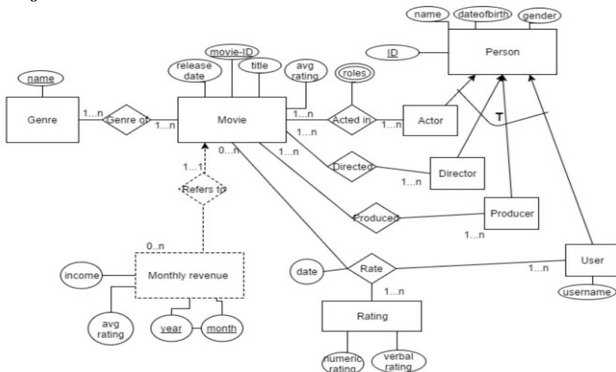
Figure.7 ER diagram
